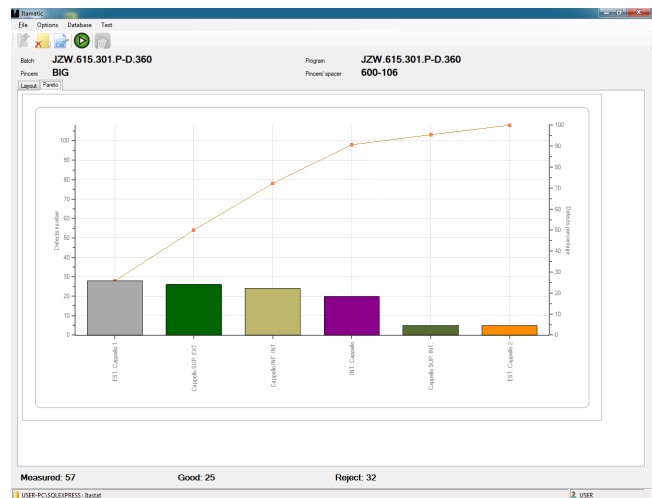
Pareto scarti
